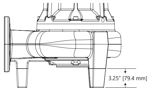
Figure 2. Point de coupe pompes 7,5–10 hp
