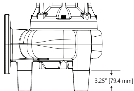
Figure 1. Point de coupe pompes 3–5 hp
